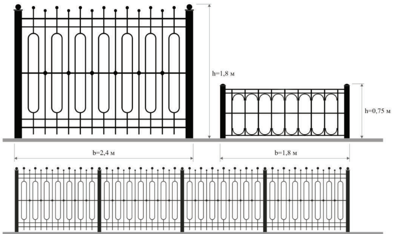
Тип ограждения № 3
