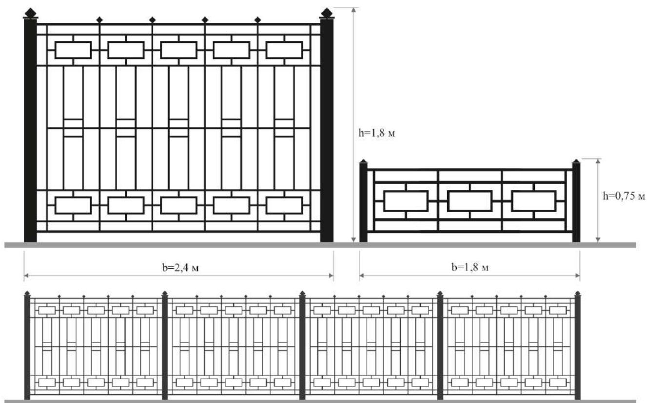
Тип ограждения № 2
