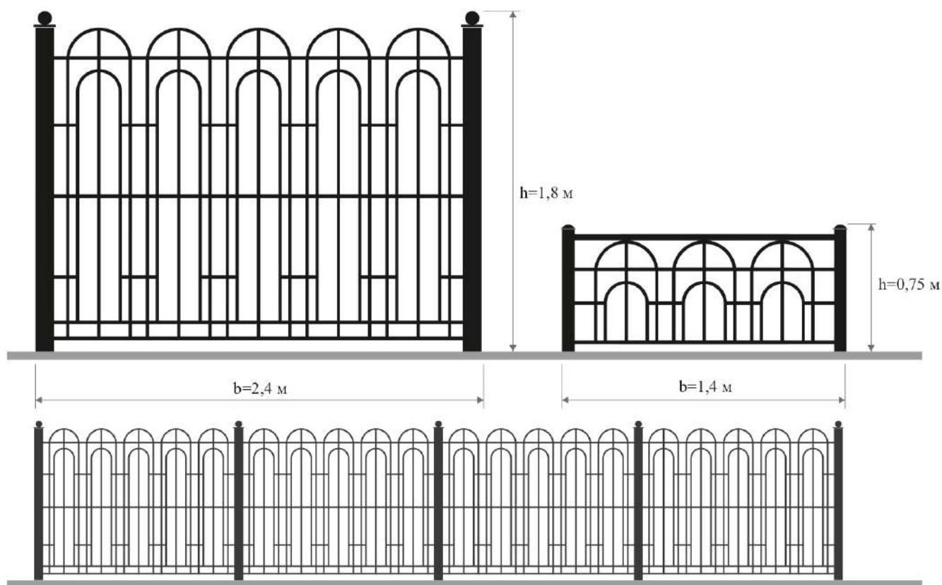
Тип ограждения № 1
